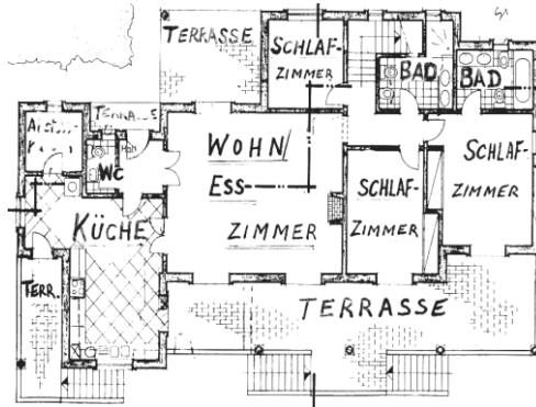
- Grundriss der Parterre -
